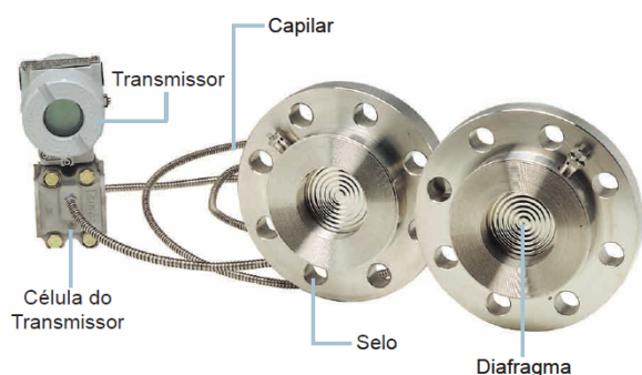
FIGURA 19 TRANSDUTOR DE PRESSÃO DIFERENCIAL COM SELO REMOTO
