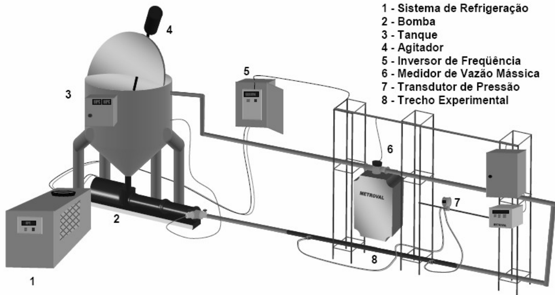
FIGURA 15 ESQUEMA DA UNIDADE DE ESCOAMENTO DE PASTA
